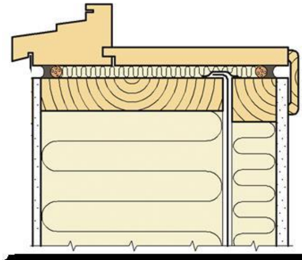
Figur 1: Principskiss av referensmodell hämtat från Byggforsk 523.701 modifierad.
