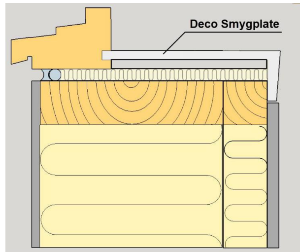
Figur 2: Principskiss av fönsterplacering med Deco Smygplatta.
